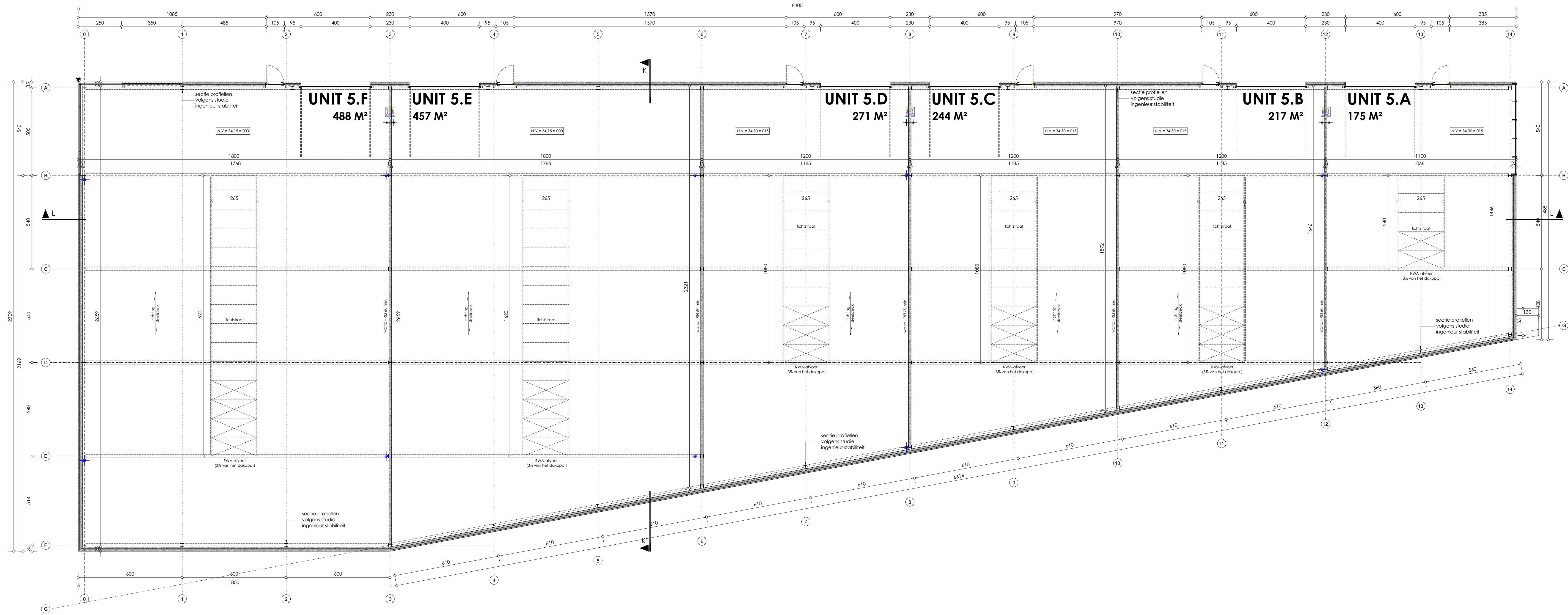
Grondplan blok 5
